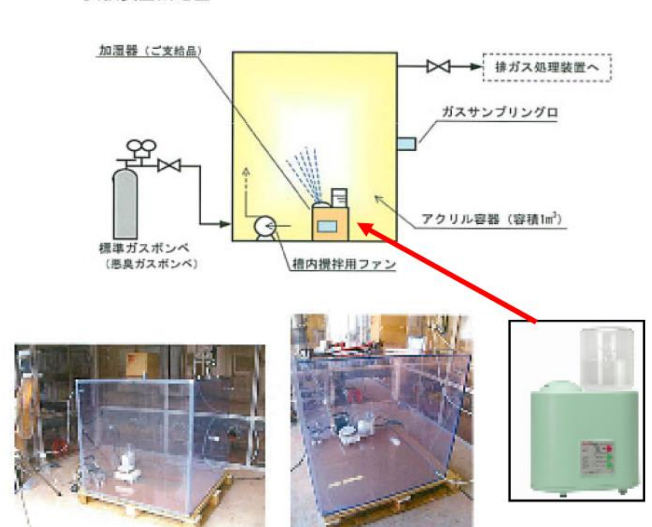
試験装置概略図
